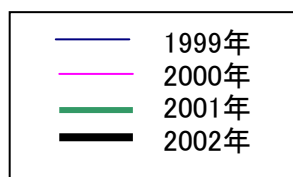
図 水温の推移(2~3m層) ※ 立神の1999年12月から2000年3月までは五ヶ所湾のデータ ※ グラフ上のデータがない部分はロガーの故障や紛失のため
